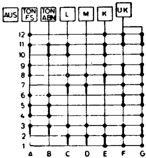
Schalterdiagramm
